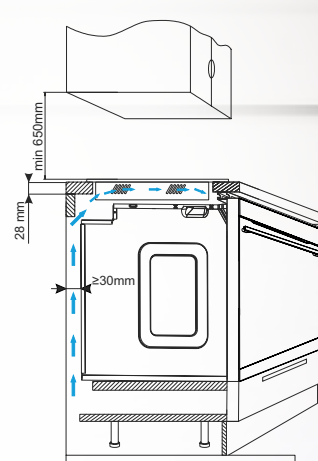
Einbau über einem Backofen
