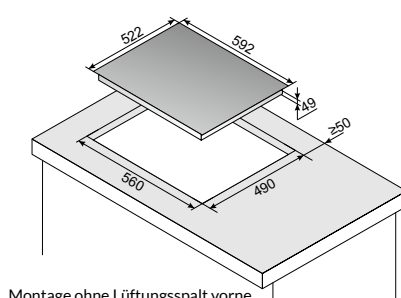
Montage ohne Lüftungsspalt vorne
