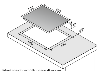
Montage ohne Lüftungsspalt vorne
