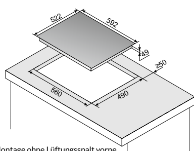
Montage ohne Lüftungsspalt vorne
